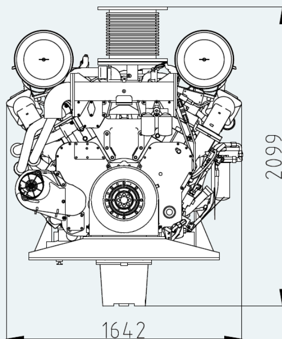
Målskisse
